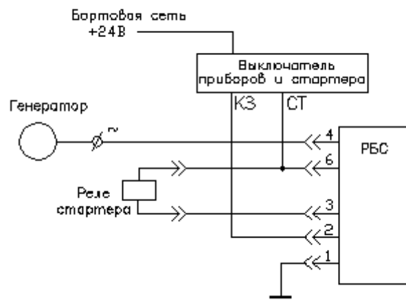
Схема электрическая подключения
